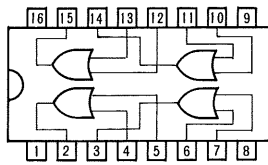
MC10103L
